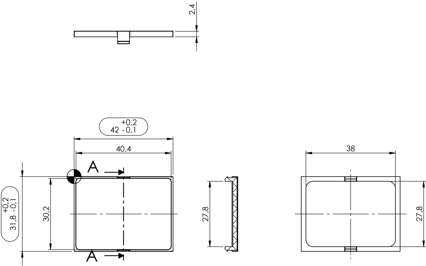
SECTION A-A
